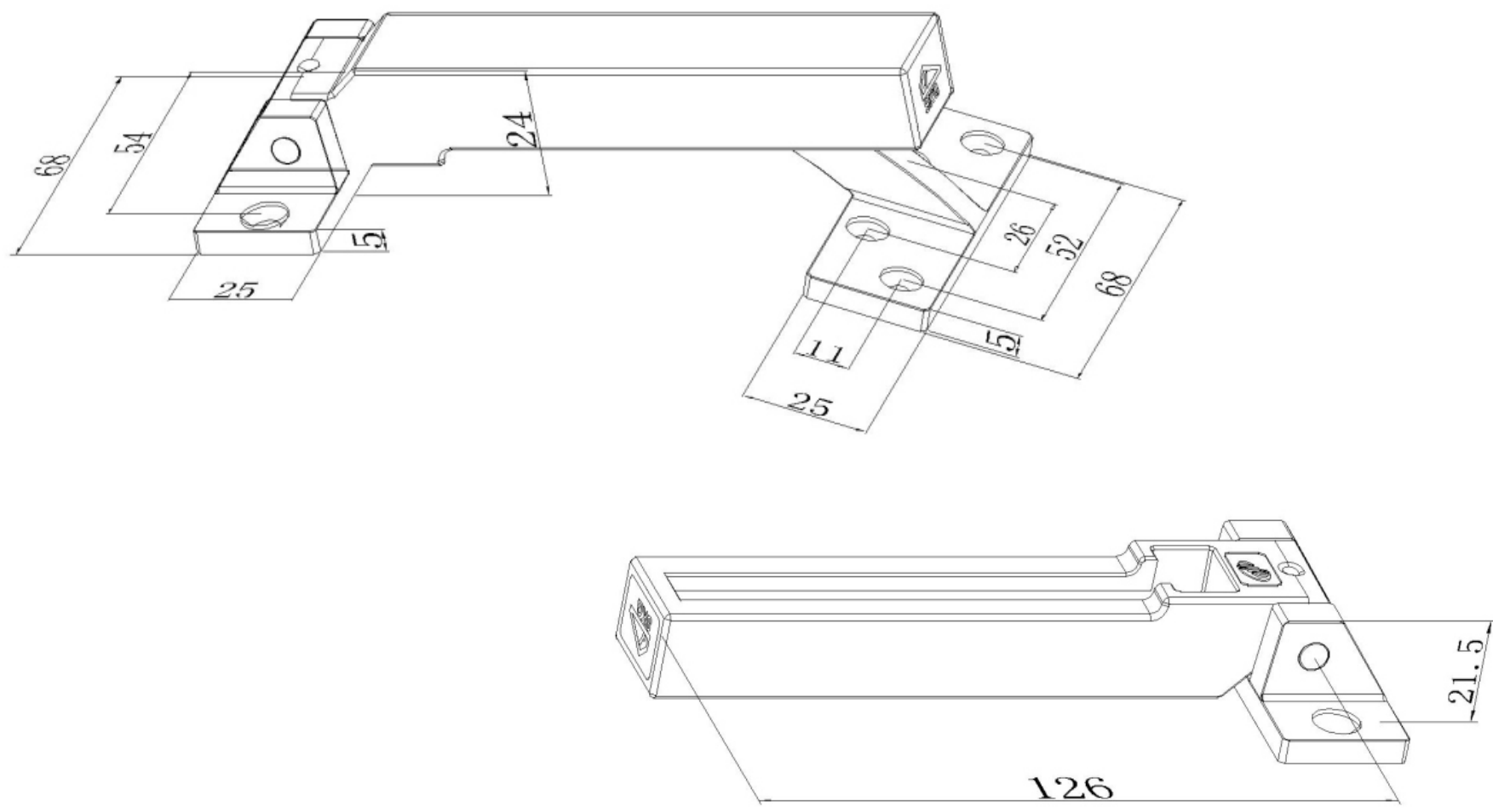
MAATVOERING KIERSTANDHOUDER ART.NR 1900.0002.04.1
