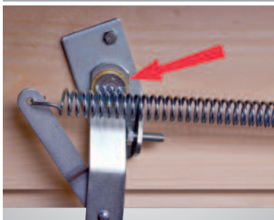
2 - hefarm met slijtvaste ring
