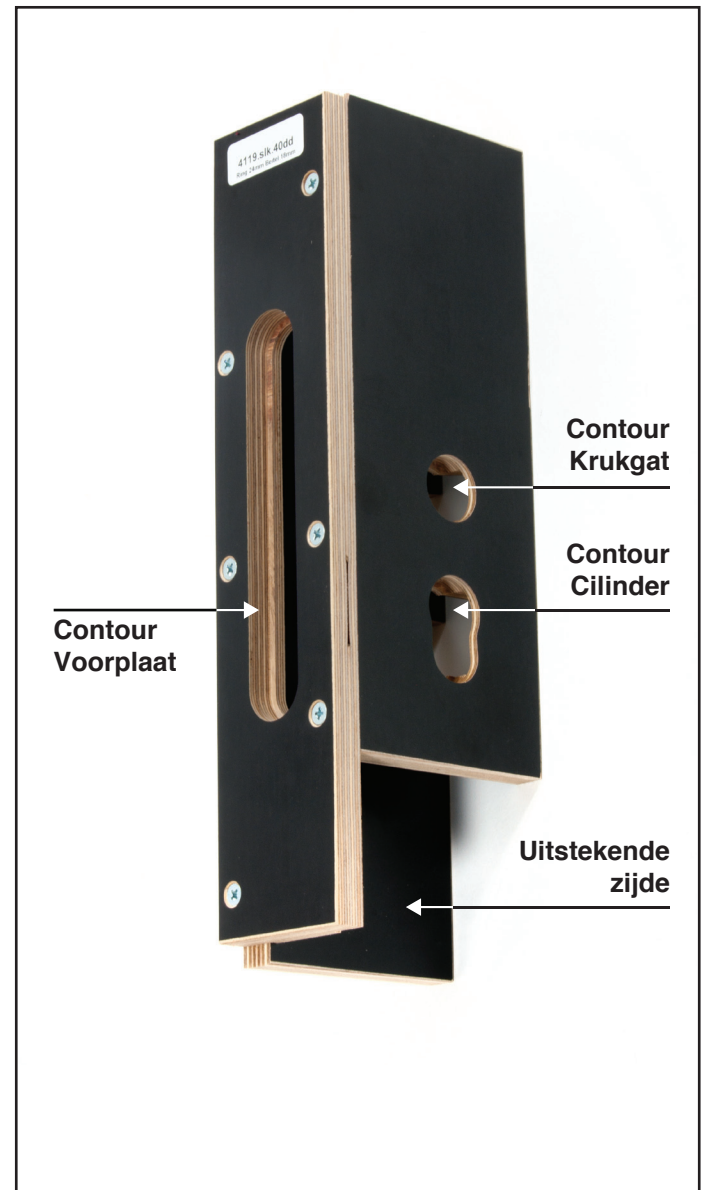
afb. 1 - Slotkast freesmal
