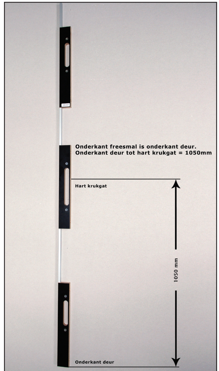
afb. 2 - Complete freesmal op strip (Lengte 2120 mm)
